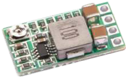
T1055 Super Mini Buck Converter DC-DC 12-24V To 5V 3A Adjustable Step Down Power Module
