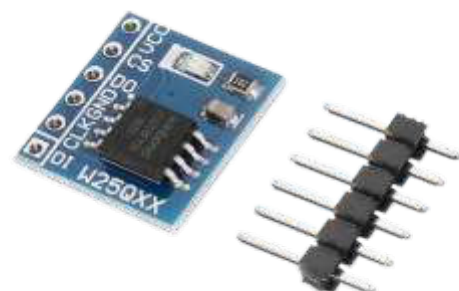
T1060 W25Q128 128Mbit 16Mbyte Capacity Flash Storage Module
